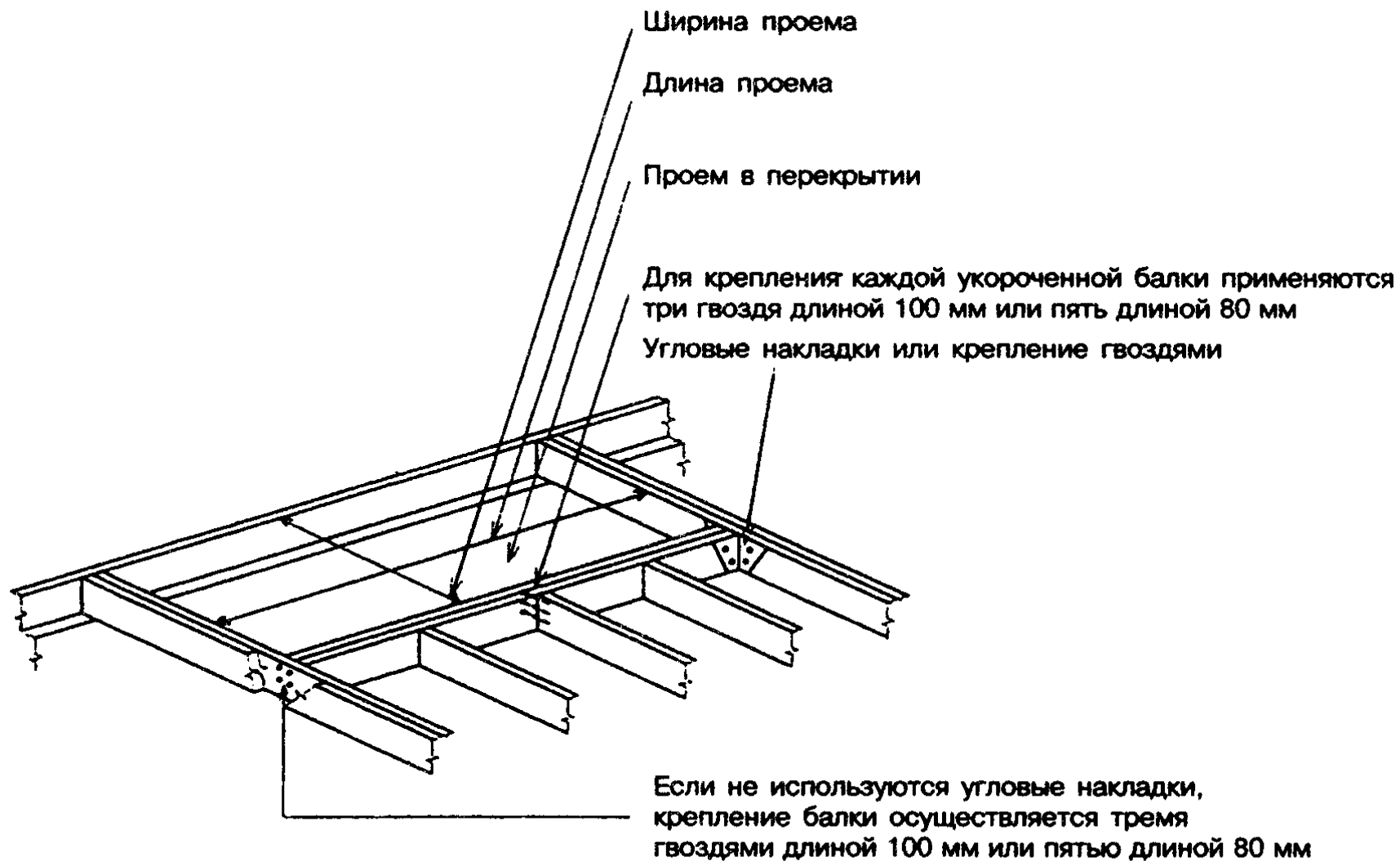
Рисунок 6-12 — Устройство проемов в перекрытии
