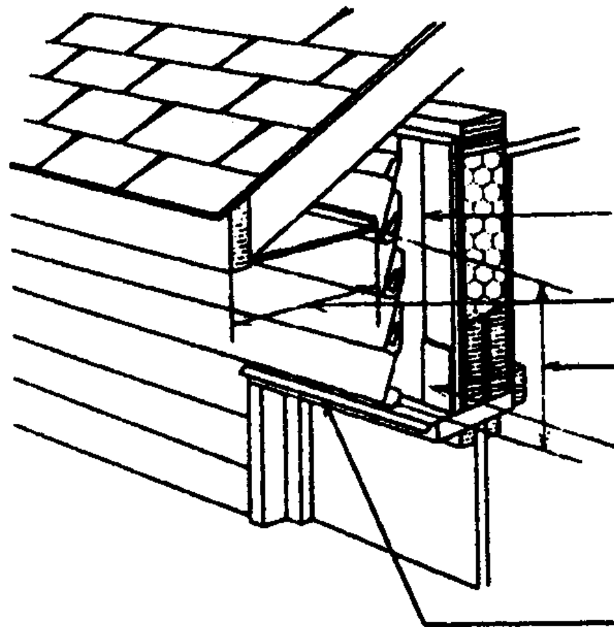
Рисунок 10-4 — Фартук над оконным (дверным) проемом
