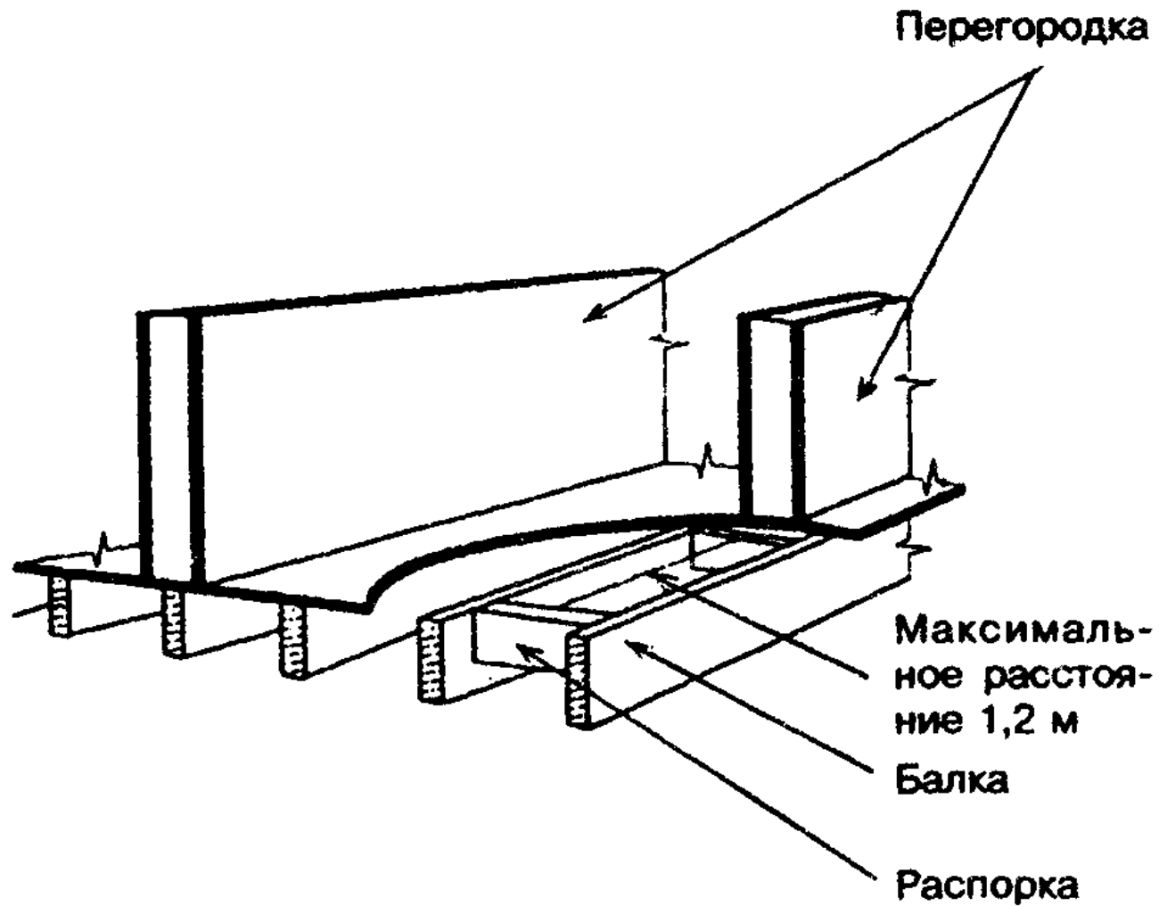
Рисунок 6-13 — Опираие перегородок
