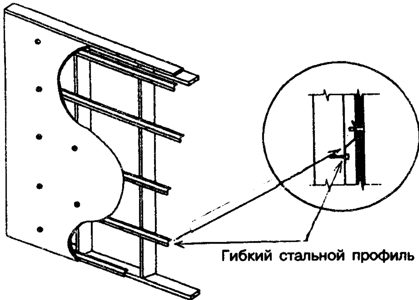
Рисунок 7-8 — Крепление обшивки каркаса для обеспечения звукоизоляции
