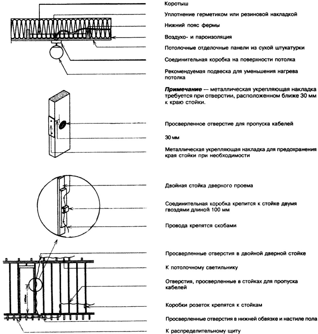
Рисунок 13-9 — Прокладка электрических проводок в элементах каркаса
