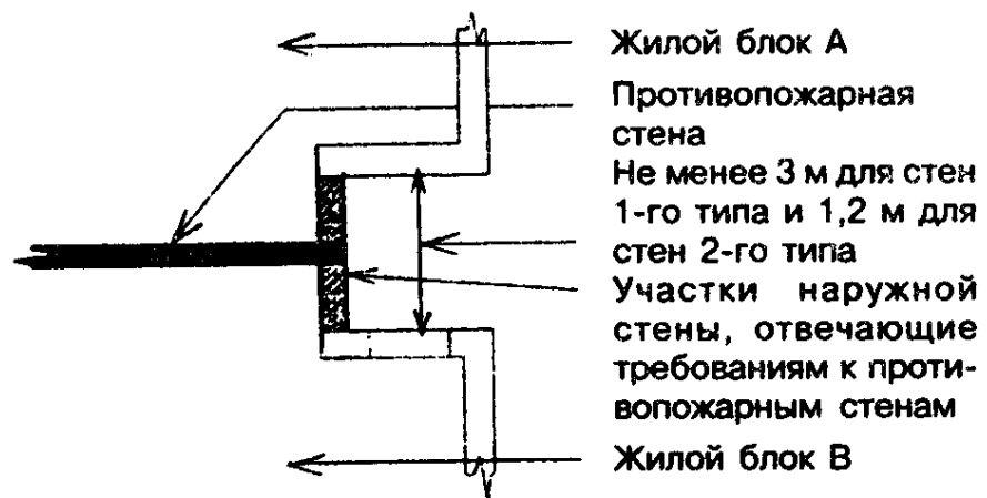
Рисунок 7-7 — Варианты устройства противопожарной стены в местах примыкания соседних блоков
