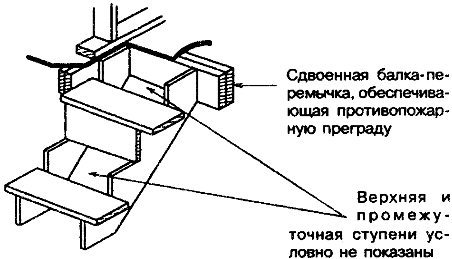
Рисунок 12-2 — Противопожарная преграда в лестничном проеме
