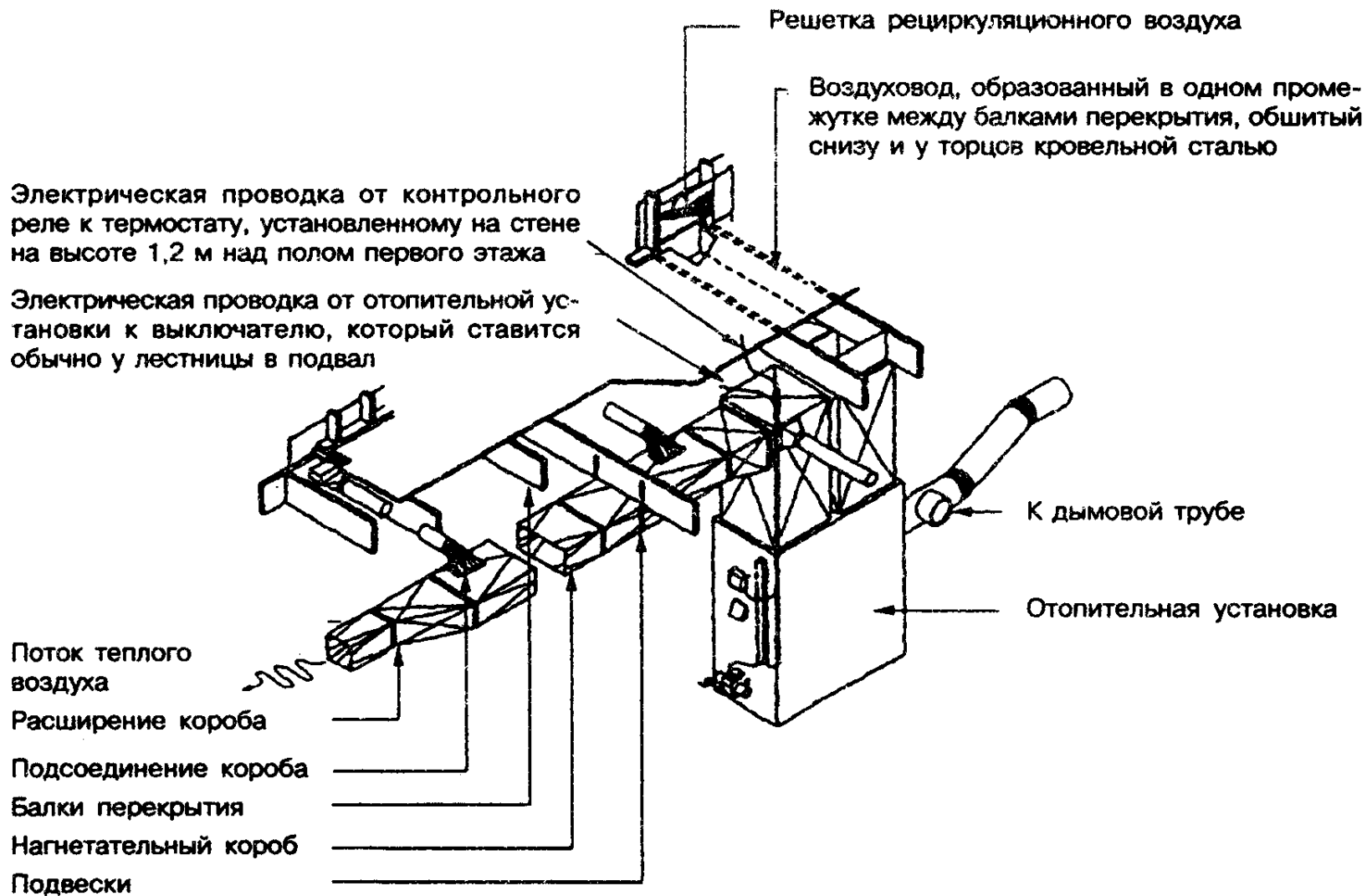
Рисунок 13-4 — Крепление воздуховодов
