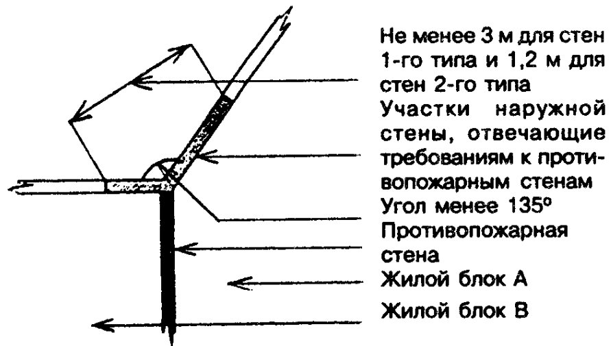
"Рисунок 7-6 - Межквартирная противопожарная стена 2-го типа каркасной конструкции"
