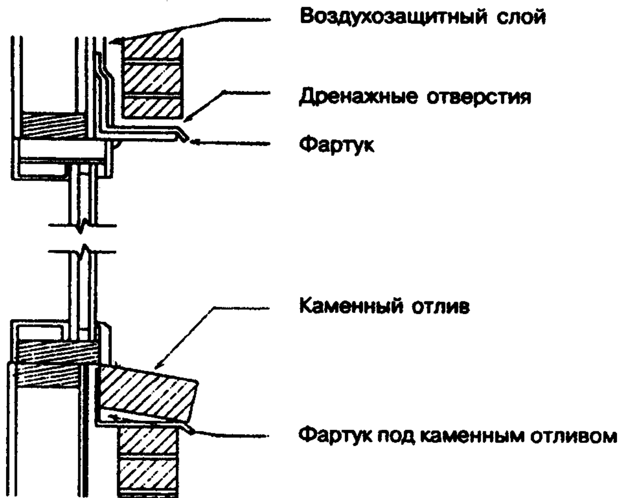
Рисунок 10-2 — Установка фартука под каменным отливом
