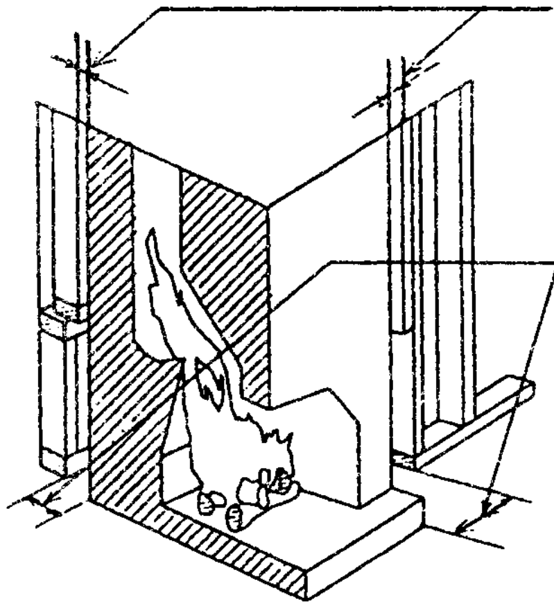
Рисунок 13-2 — Расстояние от стенок камина до каркаса здания
