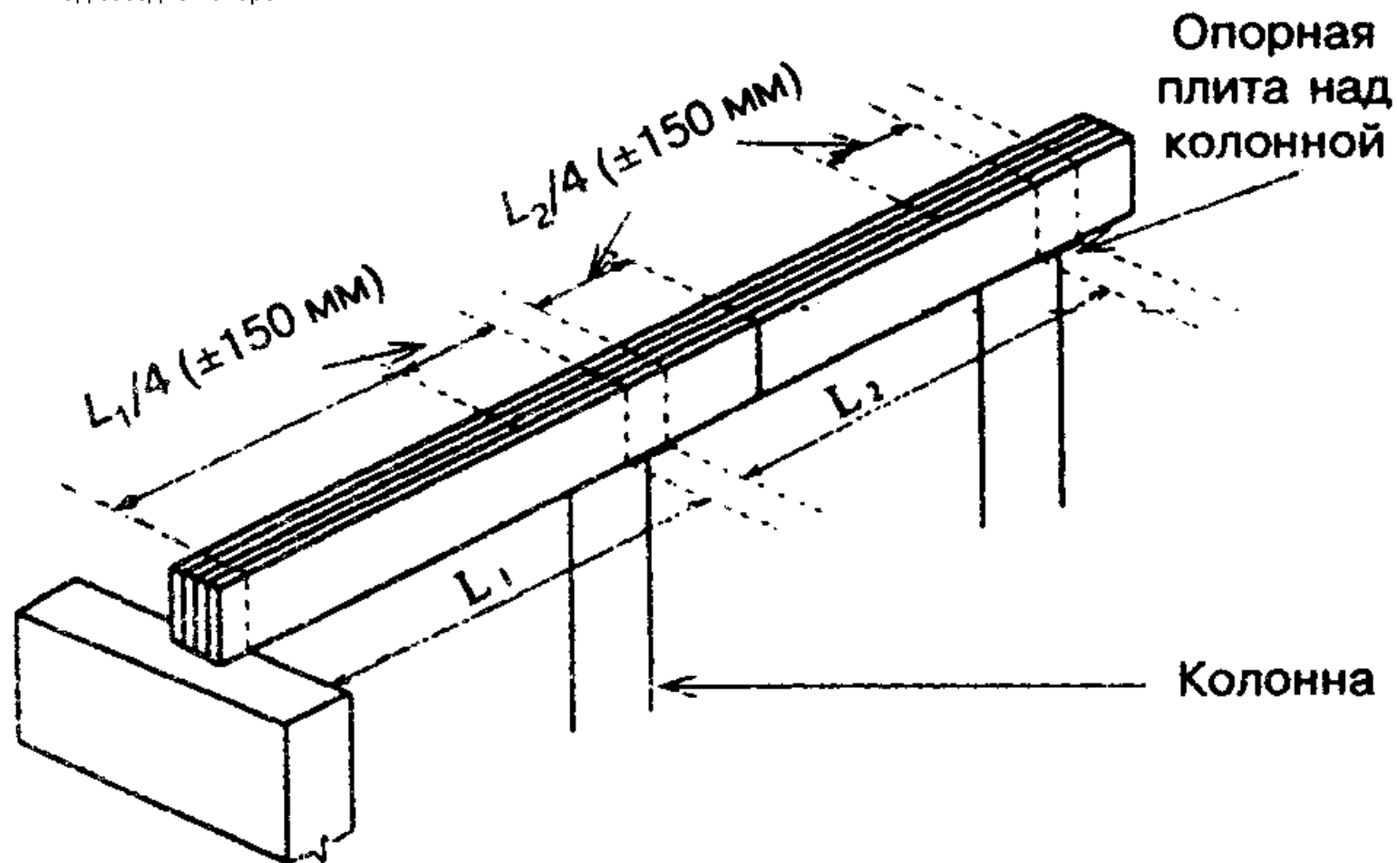
Рисунок 6-2 — Стыки досок в неразрезных прогонах составного сечения
